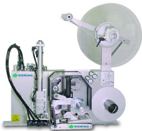
M200 Transferencia térmica de ribbon con aplicador por pistón y soplado
