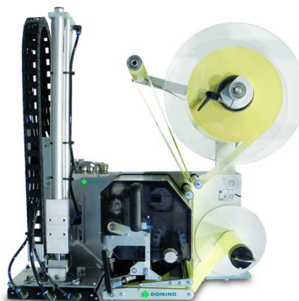
M300 Sistema de impresión y aplicación compatible con RFID
