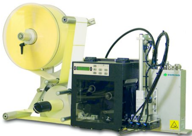
M400 Sistema de impresión OEM con aplicador por pistón y soplado
